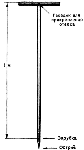
Самодельный нивелир.
