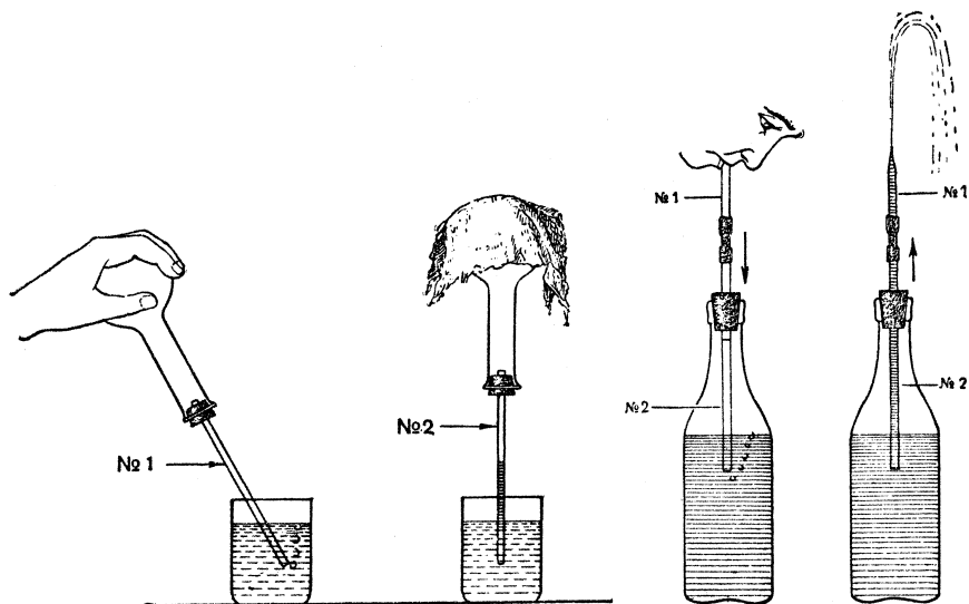
Сжимаемость и упругость воздуха.
