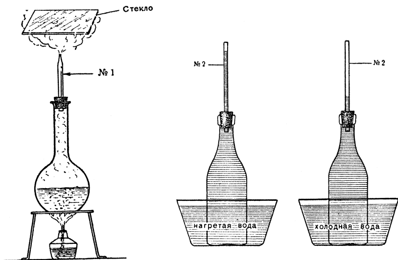
Расширение воды при нагревании и сжатие при охлаждении.
