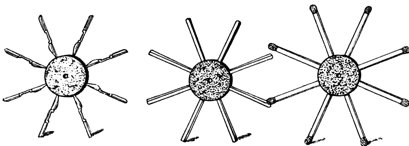
Самодельные модели водяных колёс.
