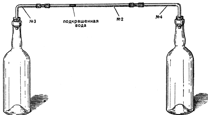
Упрощённый термоскоп.
