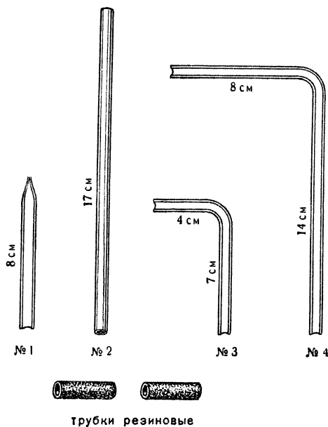
трубки резиновые
