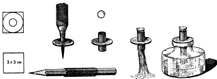
Самодельная спиртовка.
