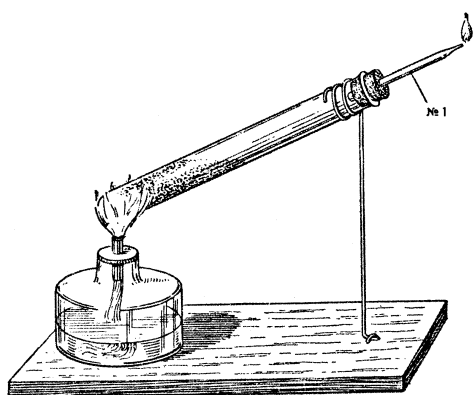
Прибор для сухой перегонки дерева
