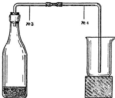
Прибор для добывания углекислого газа.
