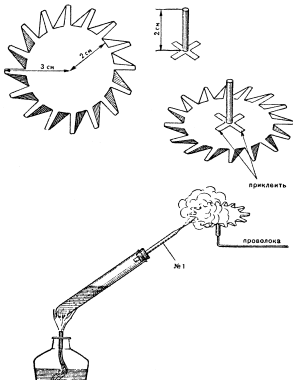
Работа пара.
