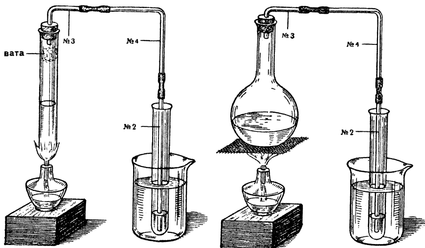
Прибор для перегонки воды.
