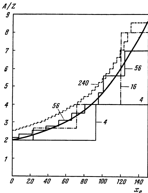
Рис. 3. Зависимость среднего значения A/Z от параметра x_e = \frac{p_e}{m_e c} . Ступенчатые линии представляют истинные значения A/Z для ядер с A=4, 16, 56 и 240. Сплошная линия дает усредненное по ядрам значение \overline{A/Z} .
