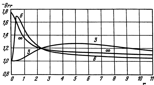
Рис. 27. Графики функции -g_{rr}(r) для ряда конфигураций из идеального газа барионов. Числа на линиях указывают значения параметра t_n(0) . По оси абсцисс отложено расстояние от центра в километрах.
