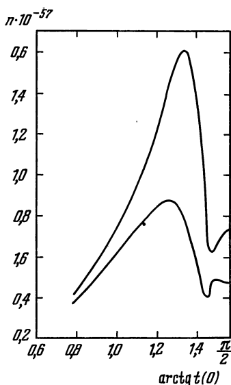
Рис. 32. Зависимость числа частиц в нейтронных звездах от параметра \arctg t_n(0) по теориям тяготения Эйнштейна (нижняя кривая) и Ньютона.
