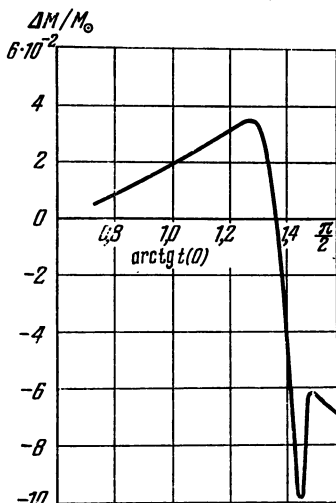
Рис. 33. Зависимость коэффициента упаковки нейтронных конфигураций от параметра \operatorname{arctg} t_n(0) по теории гравитации Эйнштейна. \Delta M = Nm_n - M — абсолютный гравитационный дефект массы.
