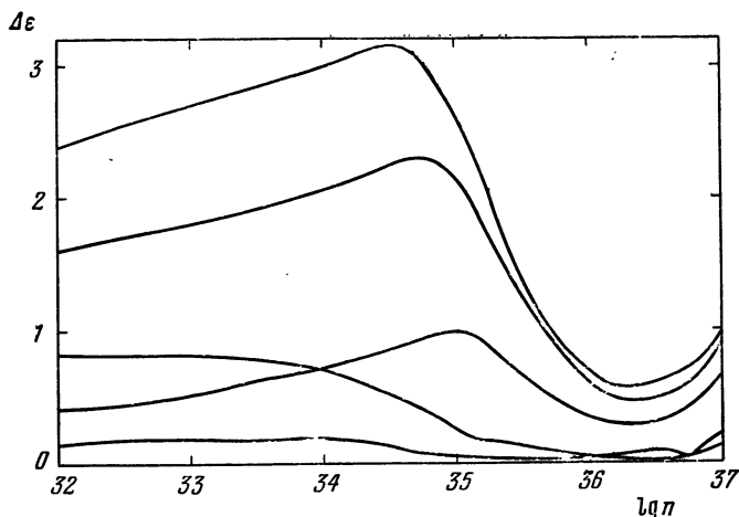
Рис. 8. По оси ординат отложена \Delta\epsilon = (\rho_A - \rho_{\min})/n , где n — плотность числа барионов, \rho_{\min} — плотность энергии в наиболее устойчивом состоянии вещества в A\epsilon и A\epsilon n -фазах. \rho_A — плотность энергии для заданного массового числа A=8, 12, 27, 125, 216 . Первые изломы (экстремумы) на линиях \Delta\epsilon(n) имеют место в точках фазового перехода A\epsilon \rightarrow A\epsilon n . Очевидно, \Delta\epsilon — разность внутренних энергий, рассчитанных на один барион. Энергия измеряется в Мэв.
