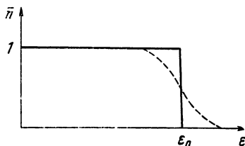
Рис. 1. Средние числа заполнения в вырожденном ферми-газе. Сплошная линия — распределение частиц при абсолютном нуле, прерывистая — при T \leq T_0 .
