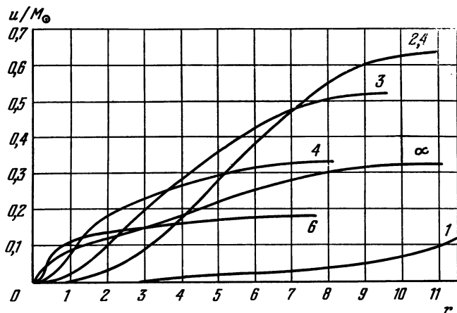
Рис. 25. Графики функции u(r) для ряда моделей барионных конфигураций (вариант идеального газа). Числами на кривых указаны значения параметра t_n(0) . Линия для модели с t_n(0)=1 продолжается до r=21,1 км. Расстояние измеряется в километрах.
