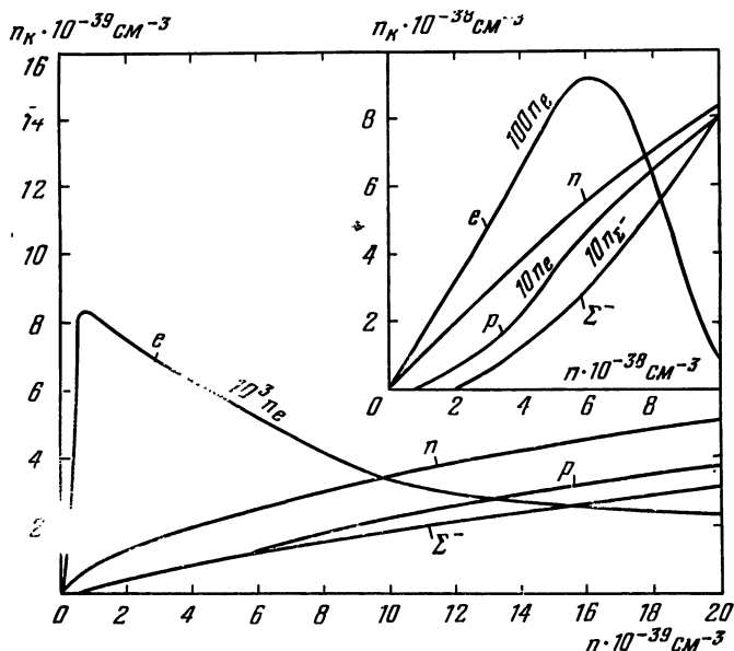
Рис. 11. Зависимость плотностей нейтронов n , протонов p , \Sigma -гиперонов и электронов e от плотности барионов. Кривые рассчитаны в предположении, что потенциальные энергии всех разновидностей одинаковы. В верхнем правом углу — те же зависимости с учетом реального ядерного потенциала.
