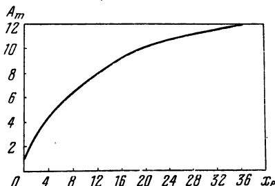
Рис. 5. Зависимость наименьшего значения массового числа ядра A_m от x_e = p_e / m_e c . Точки области, находящейся выше кривой A_m(x_e) представляют устойчивые (относительно туннельного эффекта) ядра, а под кривой — неустойчивые.
