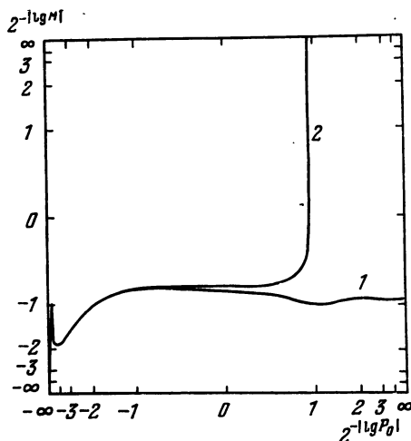
Рис. 39. Зависимость массы от центрального давления для статических конфигураций, состоящих из реального газа барионов (уравнение состояния (33.6)). По оси абсцисс отложена величина 2^{-\lg P_0} , причем она откладывается от отметки +\infty , если P \geq 1 , и от отметки -\infty , если P_0 \leq 1 . Сторона рамки принимается равной 2. По оси ординат аналогичным образом откладывается 2^{-\lg M} . По обычной теории Эйнштейна (кривая 1) масса конфигурации порядка M_\odot , а центральное давление может иметь любые значения. По релятивистской обобщенной теории (кривая 2) давление сверху ограничено, однако для массы допустимы любые значения, причем при P_0 \rightarrow 7,52 M \rightarrow \infty .
