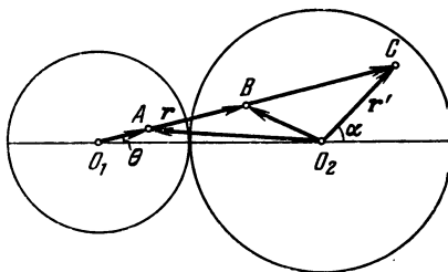
Рис. 4. К расчету туннельного эффекта. O_1O_2 = R_1 + R_2 = l , O_1C = S , O_2C = r' . А и В — некоторые точки на пути следования первого ядра по направлению O_1C , С — точка встречи двух ядер.
