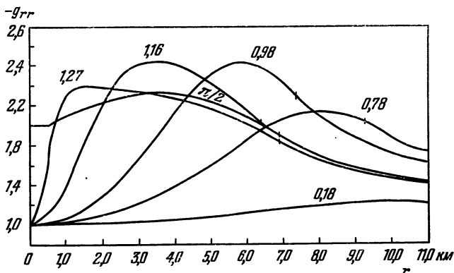
Рис. 28. Зависимость -g_{rr}(r) от r для ряда конфигураций из реального газа барионов. Над кривыми указаны значения параметра \eta = \arctg \lg \frac{\rho(0)}{\rho_1} для соответствующих конфигураций ( \rho_1 = 3,62 \cdot 10^{14} \text{ г} \cdot \text{см}^{-3} — ядерная плотность).
