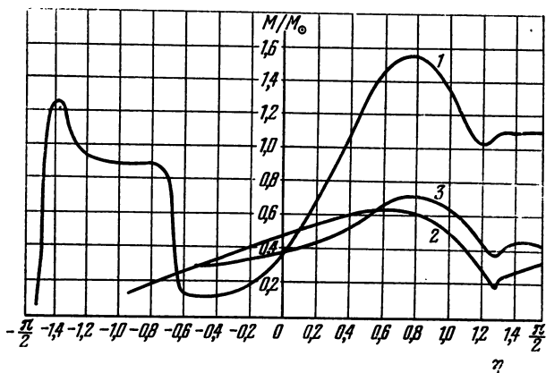
Рис. 20. Зависимость массы барионных звезд от параметра \eta = \arctg \lg \frac{\rho(0)}{\rho_1} , где \rho_1 = 3,62 \cdot 10^{14} \text{ г} \cdot \text{см}^{-3} . 1 — конфигурации, состоящие из реального газа барионов (данные таблицы 10), 2 — идеальный газ барионов, 3 — идеальный газ нейтронов. Часть кривой 1 при \eta < -0,6 представляет белые карлики.
