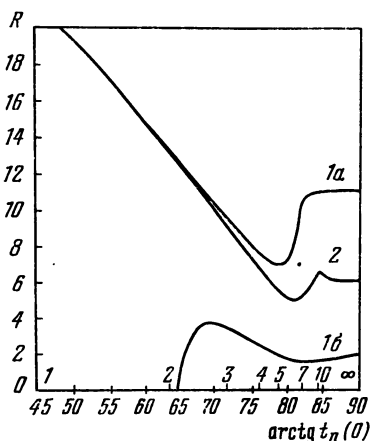
Рис. 19. Зависимость радиуса барионных звезд (кривая 1а) и их гиперонного ядра (1б) от параметра \operatorname{arctg} t_n(0) в случае идеального газа. Кривая 2 представляет радиус нейтронных конфигураций (идеальный газ). Радиус дан в километрах.
