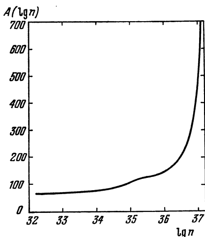
Рис. 7. Зависимость массового числа наиболее устойчивого ядра в Ae - и Aen -фазах от плотности барионов. Небольшая выпуклость при \lg n \approx 35 вызвана фазовым переходом Ae \rightarrow Aen . Перед образованием сплошного ядерного вещества, т. е. enp -фазы, наиболее устойчивыми являются ядра с A \approx 700 .
