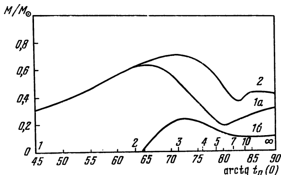
Рис. 18. Зависимость массы барионных звезд (кривая 1а) и их гиперонного ядра (кривая 1б) от параметра \operatorname{arctg} t_n(0) в случае идеального газа барионов. Кривая 2 представляет массу нейтронных конфигураций (идеальный газ).
