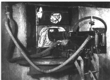
Пулеметная система со станком СТАД. Фото 1930-х гг. (РГВА)
