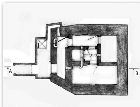
Рис. 4. План пулеметного убежища № 1005 на берегу Днестра напротив с. Меренешты.
