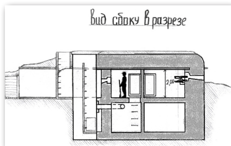
Рис. 3. Вид дота в разрезе. Рисунок автора
