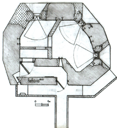
Рис. 1. План дота № 951 у с. Бычок. Рисунок автора
