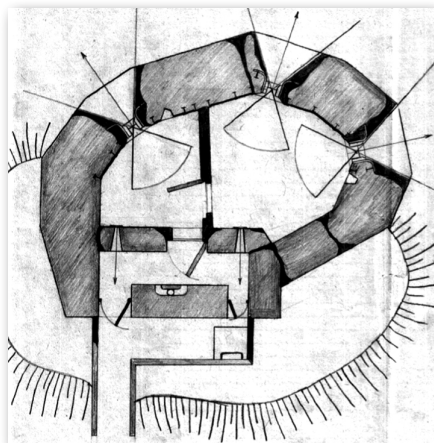
Рис. 2. План дота № 904. Рисунок автора
