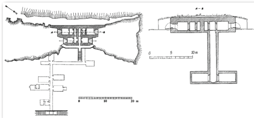
Рис. 6. План «мины» № 203 в с. Кочиеры
