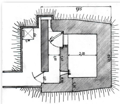
Рис. 5. План пулеметного убежища № 1051 на берегу Днестра напротив г. Бендеры. Рисунок автора
