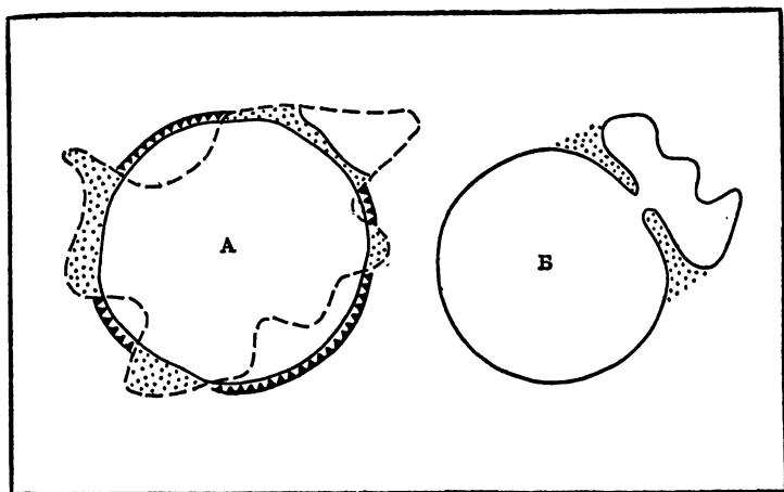
Эволюция берегов озер
