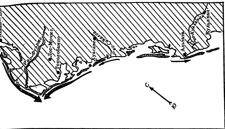
Картосхема берега Калифорнийского залива в изученном районе: 1 — разрушаемые участки берега; 2 — потоки наносов; 3 — аккумулятивные формы
