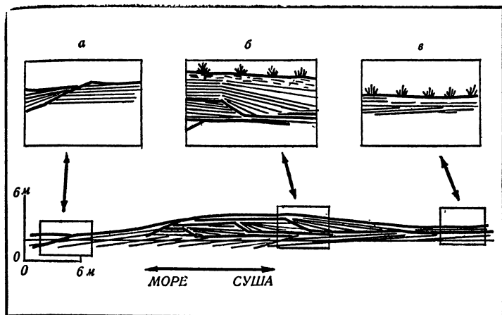
Профиль пляжевых валов (по Псути): а — зона заплеска; б — слои последовательных штормов; в — тыловая часть
