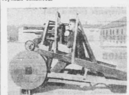
Верхние движущие колеса конструкции, насажены и сварены с осью, смещенной на 1 дюйм от центра. Большие деревянные ко-
