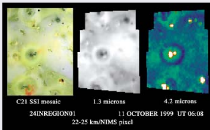
Изображение вулкана Прометей (в центре). Левый снимок сделан бортовой камерой AMC Galileo в видимом спектре, центральный и правый – в ИК-диапазоне. На правом изображении 10 ярких точек – это активные вулканы. 4 вулкана в верхней части изображения ранее были неизвестны. Четко выраженное темное кольцо вокруг Прометей – диоксид серы. Кольцо большего диаметра, чем на левом и центральном снимках. Это опровергает ранее высказанные предположения о том, что районы концентрации SO 2 на снимках в видимом диапазоне имеют белый цвет.
