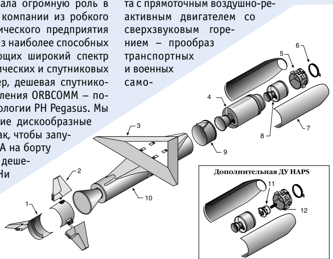
PH Pegasus XL: 1 – задняя юбка; 2 – стабилизатор; 3 – крыло; 4 – двигатель 2-й ступени; 5 – система управления; 6 – переходник ПН (Ø = 965 мм); 7 – головной обтекатель; 8 – двигатель 3-й ступени; 9 – переходник; 10 – двигатель 1-й ступени; 11 – HAPS; 12 – система отделения ДУ HAPS
