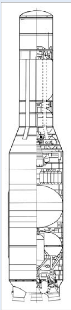
Схема РН Kistler K-1. Рисунок А.Шлядинского
