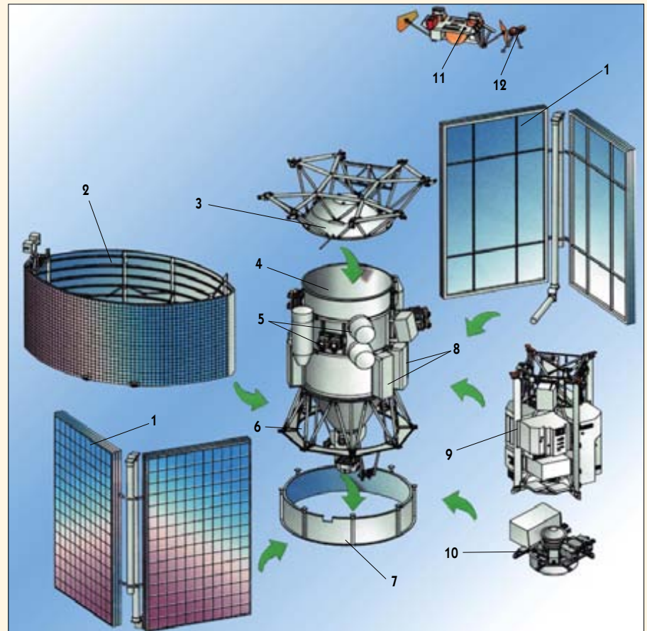
1 – пакеты панелей солнечной батареи; 2 – радиатор СТР; 3 – днище гермоконтейнера с верхней фермой; 4 – гермоконтейнер; 5 – элементы двигательной установки; 6 – опорная ферма; 7 – устройство отделения; 8 – аккумуляторная батарея; 9 – рама с приборами подсистем платформы; 10 – рама подсистемы терморегулирования; 11 – астроплата с приборами СОС; 12 – антенны КИС С-диапазона.
