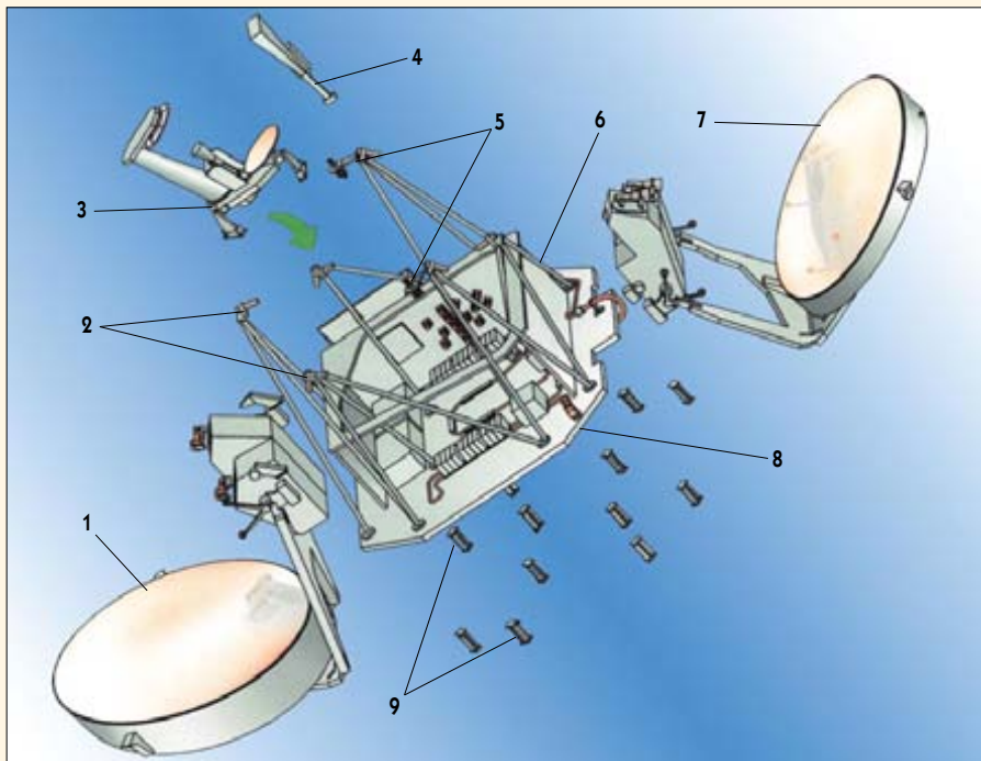
1 – приемная антенна; 2 – треножки зачекочки раскрываемых антенн; 3 – перенацеливаемая антенна Ku-диапазона; 4 – рупорная антенна KIS Ku-диапазона; 5 – антенны KIS Ku-диапазона; 6 – элементы конструкции полезной нагрузки; 7 – передающая антенна Ku-диапазона; 8 – базовая плата; 9 – опорные лезвия.
