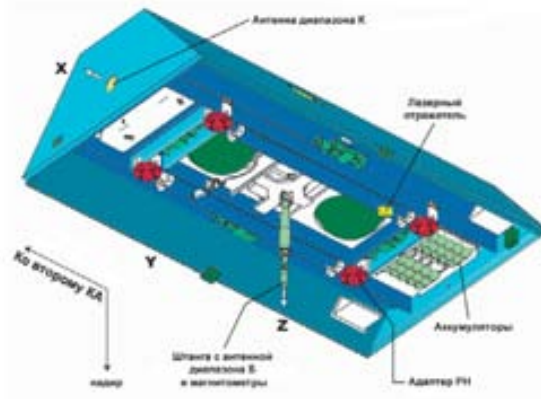
КА GRACE. Вид снизу
