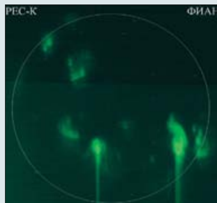
Снимок Солнца в линии 11-кратно ионизированного магния (Mg XII, длина волны 8.42Å), которой соответствует температура свыше 10 млн К
