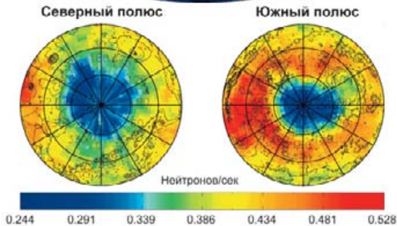
Глобальная карта нейтронного излучения Марса в диапазоне быстрых нейтронов (0.85–17 МэВ, стильбен-детектор прибора HEND, разрешение 5°x5°)
