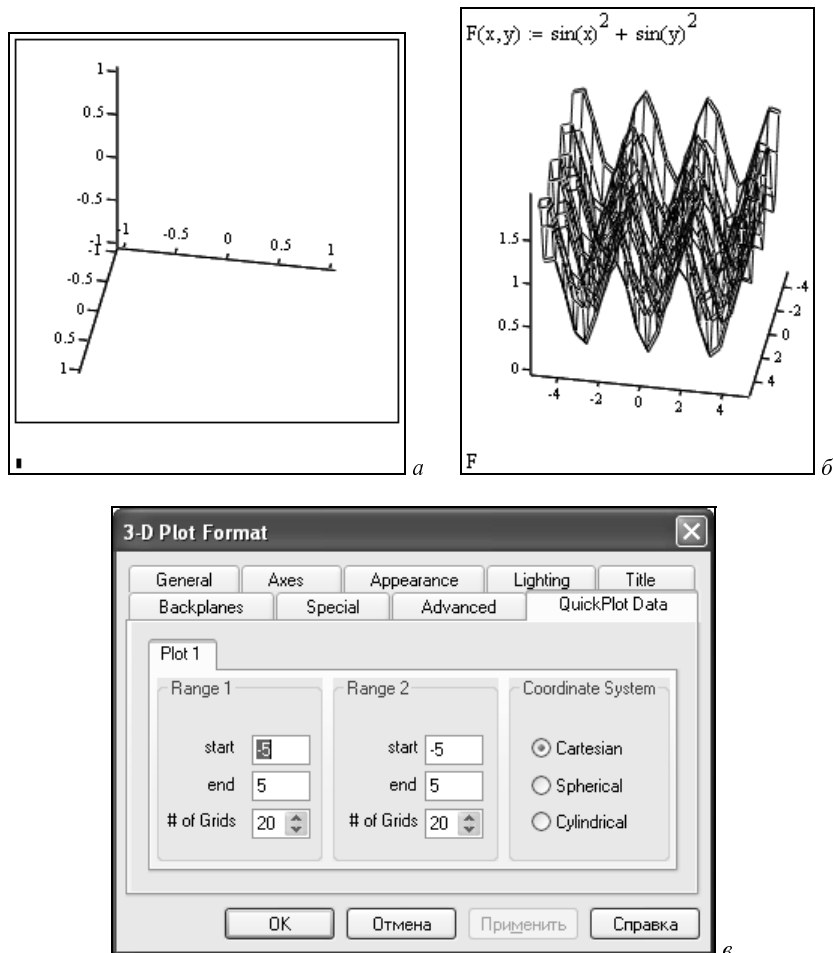
Рис. 7.11. Форматирование графика
