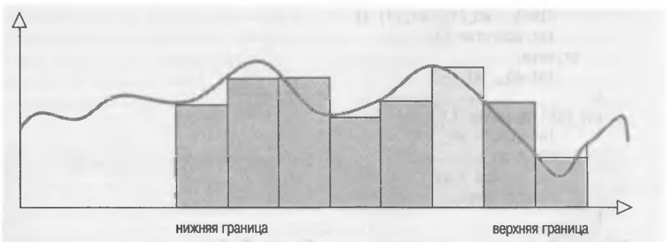
Рис. 18.1. Численное интегрирование путем суммирования площадей прямоугольников (упрощенное)
