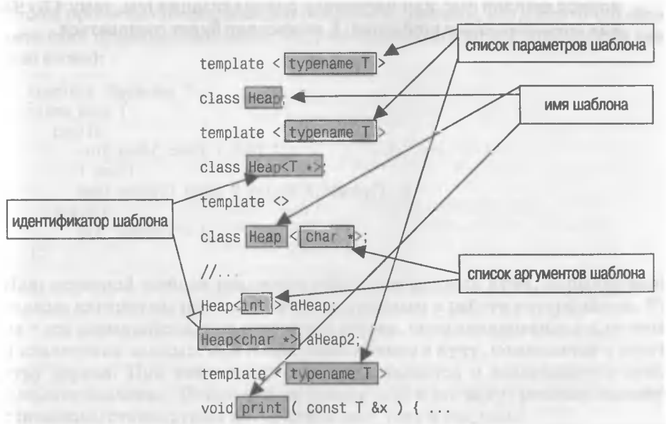
Рис. 45.1. Терминология шаблонов. Строгое соблюдение терминологии исключительно важно для точности передачи конструкции шаблона
