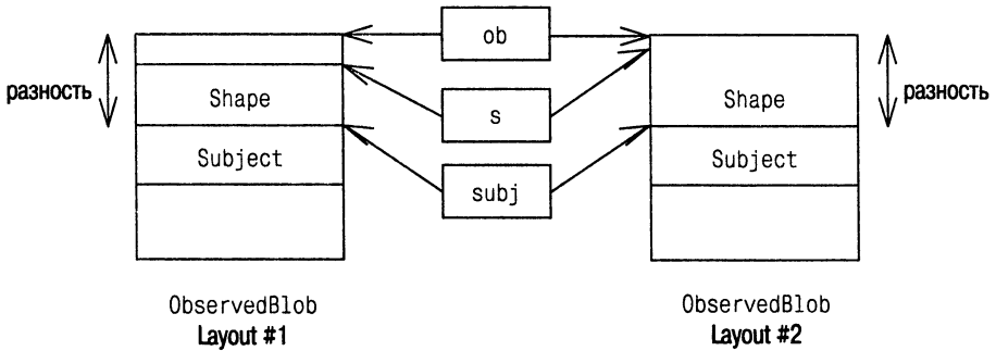
Рис. 28.1. Два возможных размещения объекта при множественном наследовании. При любом размещении объект имеет несколько адресов
