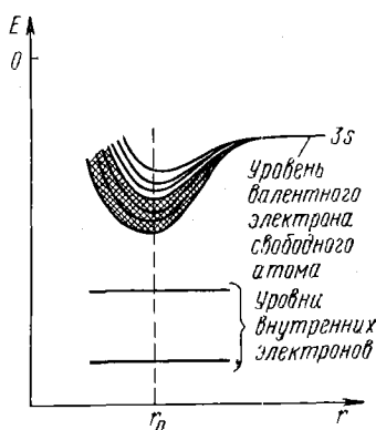
Рис. 148. Образование энергетической зоны натрия
