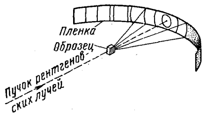
Рис. 130. Схема снятия дебаграммы
