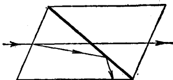
Рис. 164. Призма Николя
