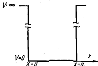
Рис. 10. Одномерный потенциальный ящик
