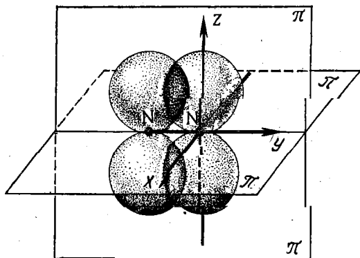
Рис. 79. Схема, показывающая образование химических связей в молекуле N_2
