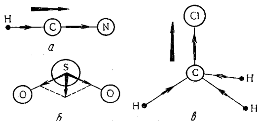
Рис. 62. Сложение дипольных моментов связей в молекулах: а — HCN; б — SO_2 ; в — CH_3Cl
