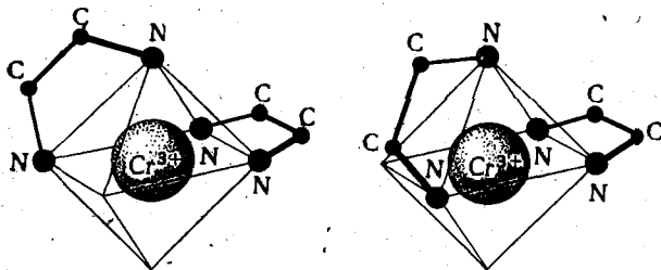
Рис. 100. Схематическое изображение структур зеркальных изомеров комплексов хрома с этилендиаминном. Атомы водорода в молекуле этилендиамина не показаны
