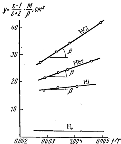
Рис. 60. График для определения дипольного момента ( \mu = 0,01282 \times 10^{-18} \sqrt{\text{tg} \beta} )
