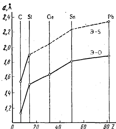
Рис. 28. Зависимость расстояний Э—S и Э—O от порядкового номера элемента
