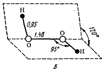
Рис. 44. Строение молекул: а — ацетилена; б — перекиси водорода (над связями указаны межатомные расстояния)
