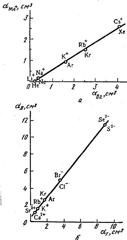
Рис. 98. Сравнение поляризуемостей: а — атомов благородных газов и ионов щелочных металлов; б — двух рядов изоэлектронных ионов
