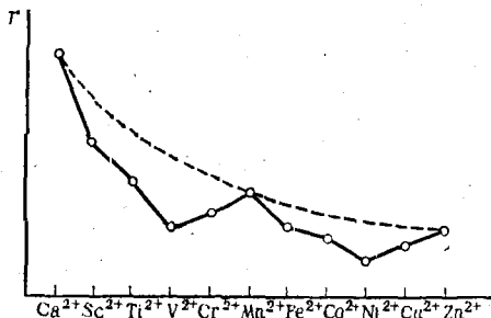
Рис. 105. Изменение радиусов ионов в ряду \text{Ca}^{2+} - \text{Zn}^{2+}
