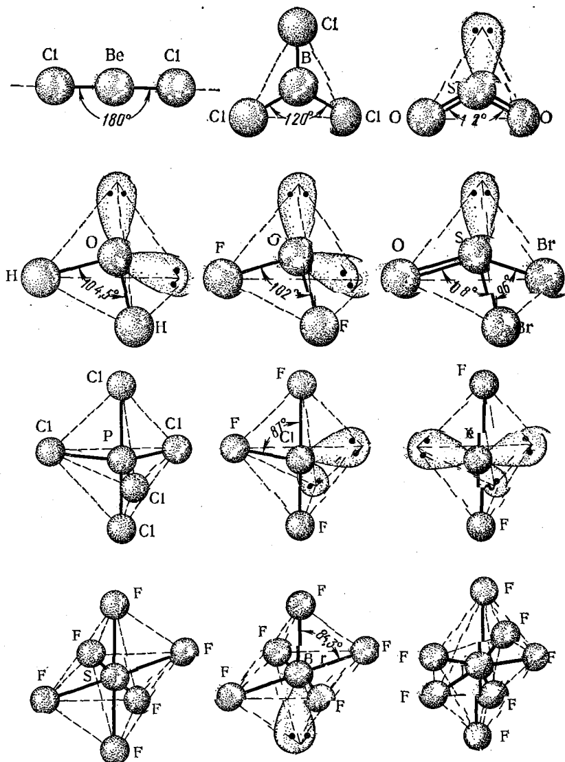
Рис. 47. Объяснение конфигурации различных молекул с помощью модели отталкивания электронных пар
