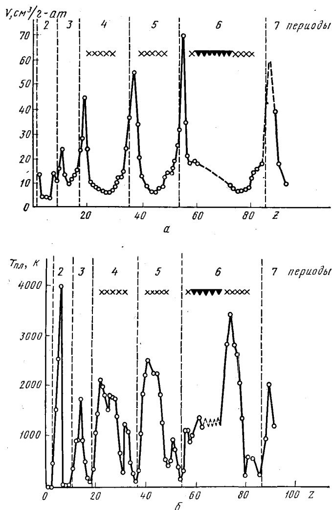
Рис. 24. Зависимость от порядкового номера элемента а — атомного объема простых веществ; б — их температуры плавления;
