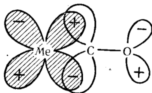
Рис. 110. Схема, показывающая образование \pi -связи между атомом металла и молекулой CO
