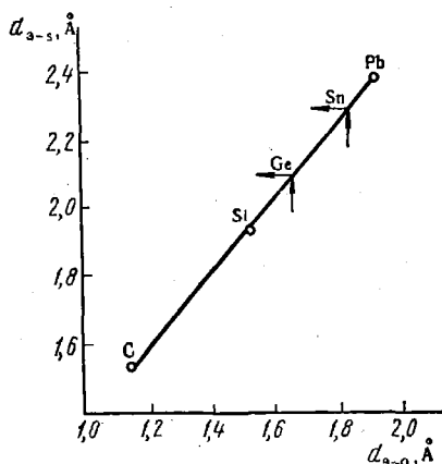
Рис. 29. Взаимосвязь межатомных расстояний Э—O и Э—S
