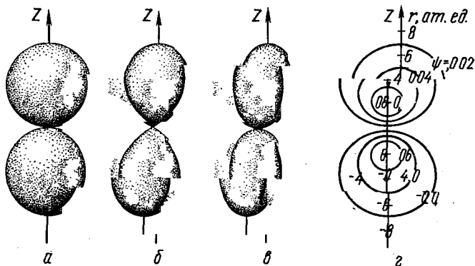
Рис. 19. Изображение 2p_z -орбитали:
