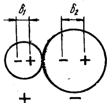
Рис. 97. Взаимная поляризация ионов
