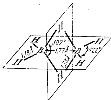
Рис. 87. Строение диборана
