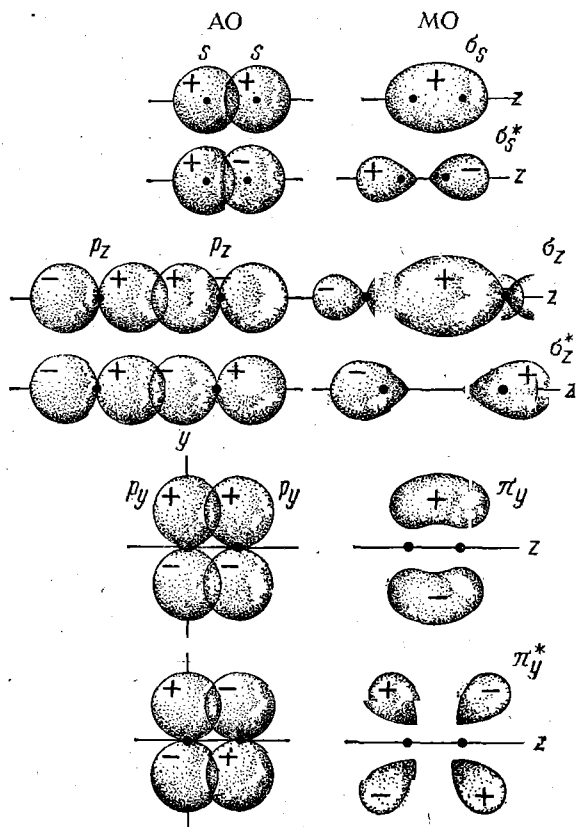
Рис. 89. Образование молекулярных орбиталей из атомных
