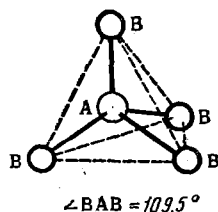
Рис. 45. Варианты строения молекулы \text{AB}_4
