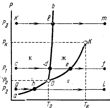
Рис. 116. Диаграмма состояния однокомпонентной системы
