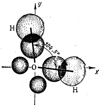
Рис. 71. Перекрывание волновых функций электронов при образовании молекулы H_2O
