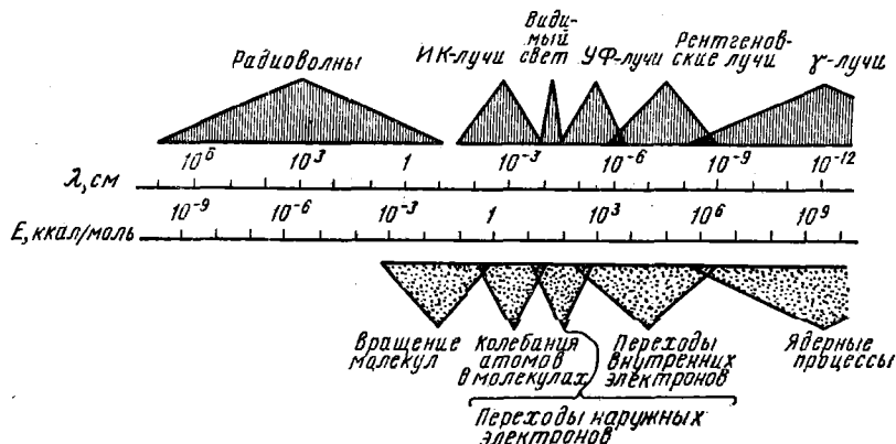
Рис. 159. Длины волн и энергии различных видов электромагнитного излучения
