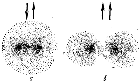
Рис. 69. Электронные облака атомов водорода при различной взаимной ориентации спинов электронов:
