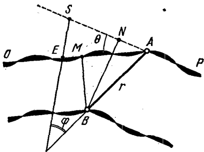
Рис. 165. Рассеяние волн молекулой
