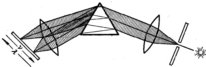
Рис. 3. Схема действия спектроскопа
