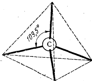
Рис. 38. Расположение валентностей атома углерода в пространстве
