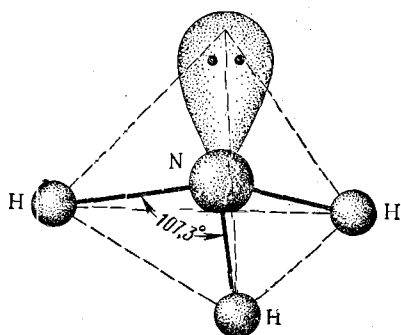
Рис. 46. Объяснение конфигурации молекулы \text{NH}_3
