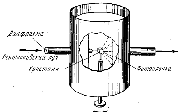
Рис. 129. Схематическое изображение камеры для получения рентгенограмм по методу вращения кристалла
