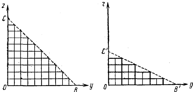
Рис. 120. Иллюстрация закона целых чисел. Отрезки OC и OC' , отсекаемые на оси z гранями CB и C'B' , относятся как 2 : 1
