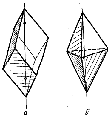
Рис. 125. Фигуры, обладающие зеркально-поворотной (а) и инверсионной (б) осью
