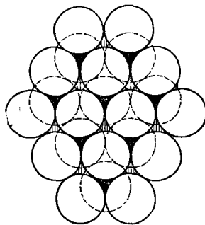
Рис. 134. Плотная упаковка двух слоев шаров
