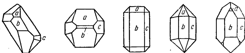
Рис. 118. Различные формы кристаллов кварца
