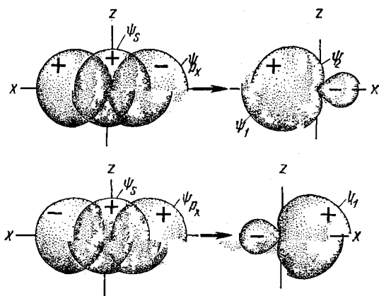
Рис. 73. Образование sp -гибридных орбиталей из s - и p -орбиталей
