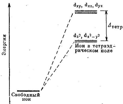
Рис. 104. Расщепление энергетических уровней d -электронов в тетраэдрическом поле
