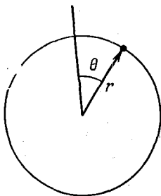
Рис. 14. Одномерный жесткий ротатор
