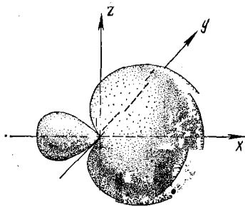
Рис. 74. Поверхность гибридной волновой функции
