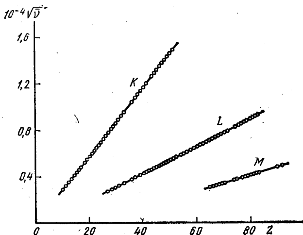
Рис. 26. Зависимость \sqrt{D} для линий рентгеновского спектра от порядкового номера элемента
