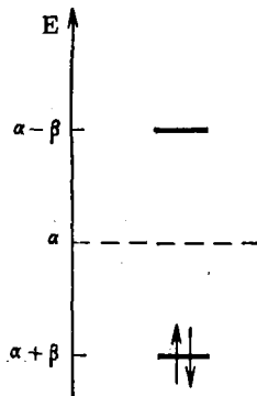
Рис. 92. Уровни энергии \pi -электронов в этилене
