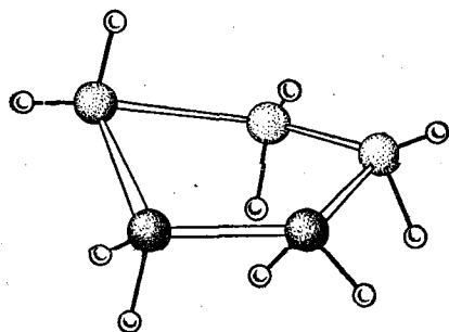
Рис. 49. Строение молекулы цикlopентана
