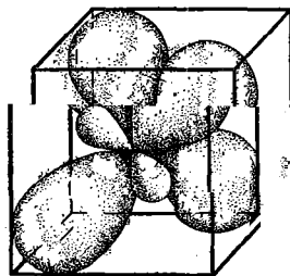
Рис. 75. Пространственное расположение гибридных электронных облаков атома углерода
