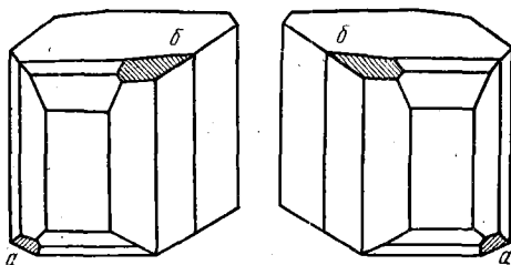
Рис. 40. Кристаллы зеркальных изомеров натриево-аммонийной соли винной кислоты.
