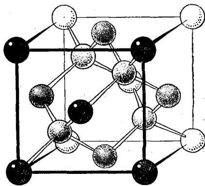
Рис. 138. Структура алмаза
