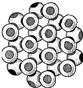
Рис. 141. Структура льда
