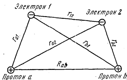
Рис. 67. Расстояния между частицами в молекуле водорода
