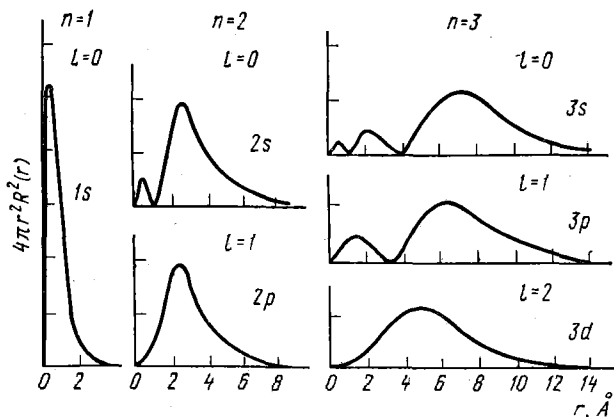
Рис. 17. Радиальное распределение вероятности нахождения электрона для различных состояний атома водорода
