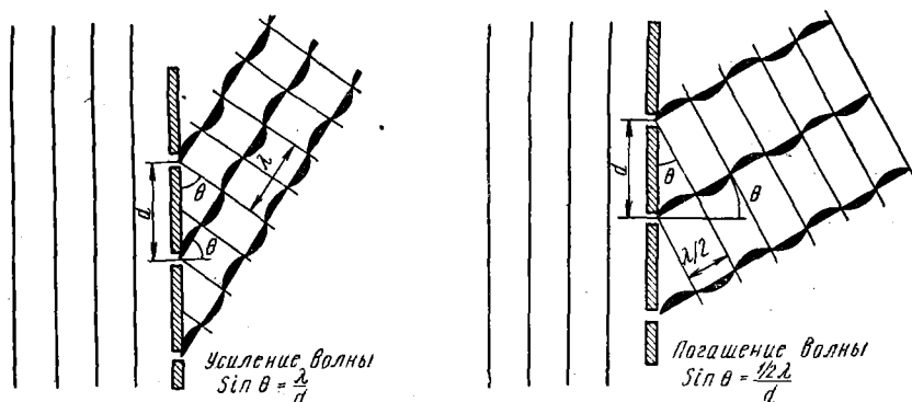
Рис. 161. Интерференция волн при прохождении через дифракционную решетку
