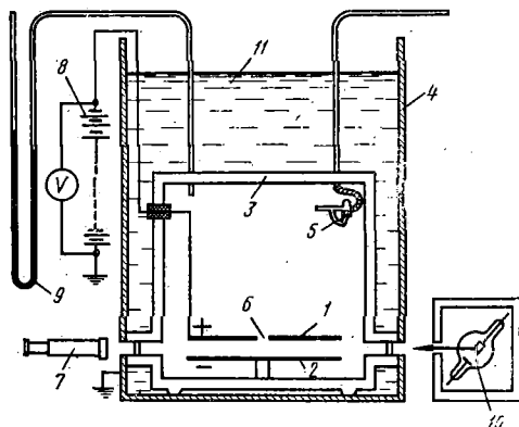
Рис. 1. Схематическое изображение установки Миллика для измерения заряда электрона:
