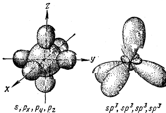
Рис. 76. Схема, показывающая перераспределение электронной плотности при образовании гибридных орбиталей
