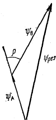
Рис. 166. Векторное сложение амплитуд
