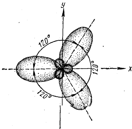
Рис. 78. Расположение электронных облаков при sp^2 -гибридизации
