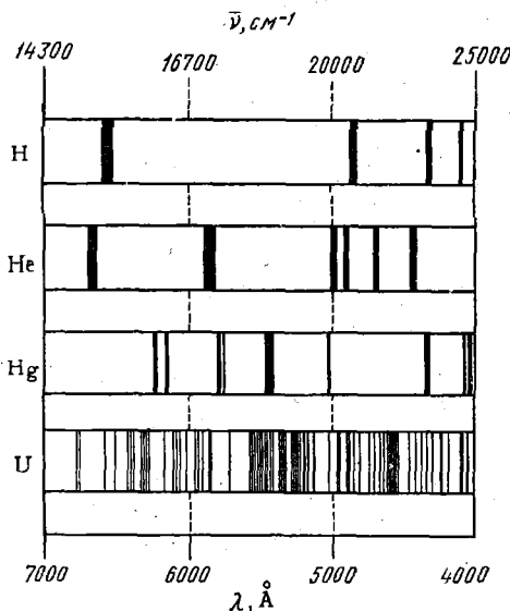
Рис. 4. Схематическое изображение спектров некоторых элементов.
