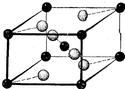
Рис. 143. Структура рутила.
