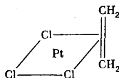
Рис. 111. Строение иона [\text{Pt}(\text{C}_2\text{H}_4)\text{Cl}_3]^-
