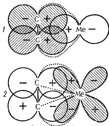
Рис. 112. Схема, показывающая образование связей в \pi -комплексе: 1 — образование связи в результате перекрывания связывающей \pi -МО лиганда и d -орбитали металла; 2 — образование связи при перекрывании разрыхляющей \pi -МО лиганда и d -орбитали металла
