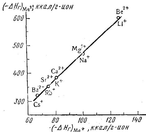
Рис. 154. Взаимосвязь теплот гидратации катионов \text{Me}^+ и \text{Me}^{2+}
