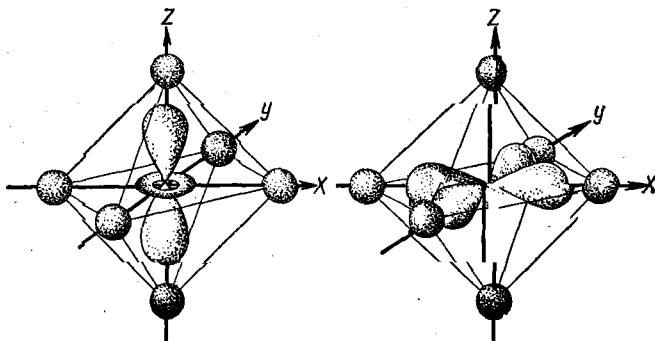
Рис. 101. Орбитали d_{z^2} и d_{x^2-y^2} в октаэдрическом поле
