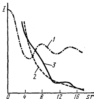
Рис. 167. Распределение интенсивности потока электронов, рассеянных молекулами \text{Br}_2 :
