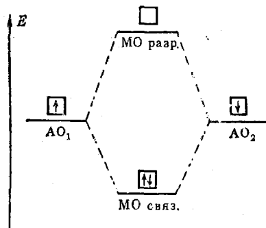
Рис. 88. Образование молекулярных уровней энергии из атомных
