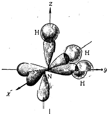
Рис. 72. Схема перекрывания электронных облаков при образовании молекулы NH_3
