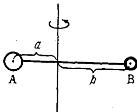
Рис. 169. Вращение двухатомной молекулы
