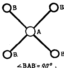
Рис. 45. Варианты строения молекулы \text{AB}_4
