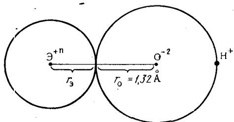
Рис. 36. Схема Косселя
