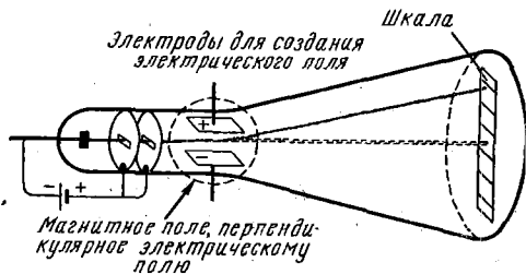
Рис. 2. Схематическое изображение прибора для определения величины e/m для электронов
