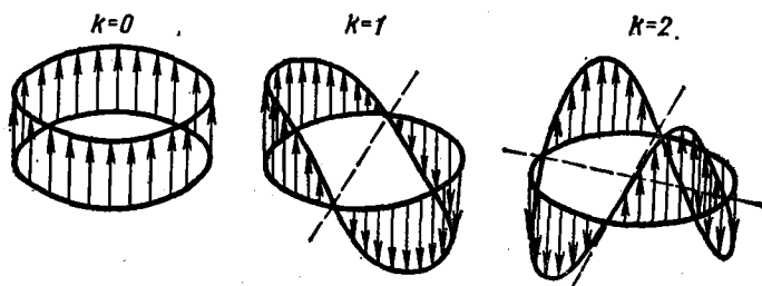
Рис. 15. Графическое изображение волновых функций для одномерного жесткого ротатора
