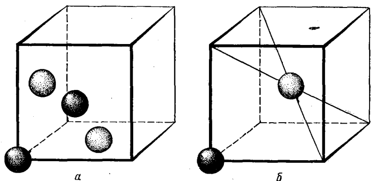
Рис. 132. Элементарная ячейка кристаллической решетки: а — меди (кубическая гранецентрированная решетка); б — натрия (кубическая объемноцентрированная решетка)
