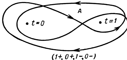
Рис. 4. Области сходимости.
