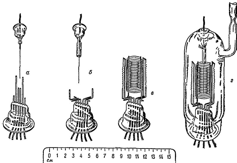
Рис. 1. Ионизационный манометр.
