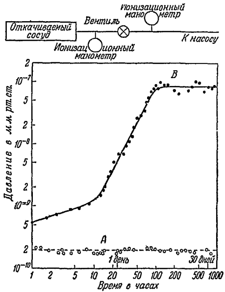
Рис. 3. Насыщение ионизационного манометра.
