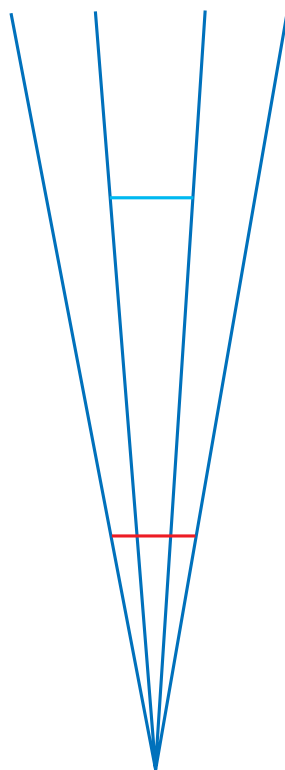
Рис. 3. Иллюзия Понцо
