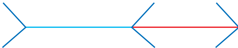
Рис. 2. Иллюзия Мюллера–Лайера
