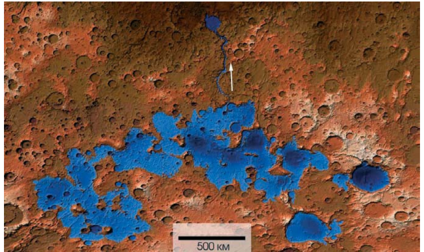
Долина Маадим в кратере Гусева (белая стрелка) могла сформироваться в результате разлива реки. Голубым показана область, в которой 3,5 млрд. лет назад, возможно, существовал грандиозный комплекс озер (по данным MOLA).
