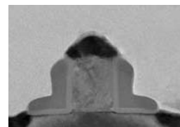
НАНОТРАНЗИСТОР первого поколения фирмы Intel.
