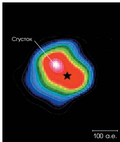
Система Веги (25 св. лет от Земли). Черной звездочкой в центре отмечено положение самой звезды. По данным компьютерного моделирования, яркий объект (левее и выше звезды) – это планета с массой, вдвое большей массы Юпитера. Изображение получено в субмиллиметровых волнах. Масса Веги, как и масса HD 141569, вдвое больше массы Солнца.
