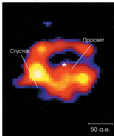
Система ε Эридана (10 св. лет от Земли). Сгустки и дыры могут быть результатом воздействия планеты с массой около массы Сатурна, движущейся по вытянутой орбите. Спектральные данные позволяют предположить существование другой планеты, находящейся ближе к звезде. Изображение получено в субмиллиметровых волнах.
