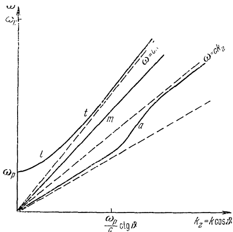
Рис. 77. То же, что и на рис. 76, но для распространения волн под углом к магнитному полю ( \vartheta \gg m_e c^2/e_* ). l — область дисперсионной кривой, где колебания продольны, t — поперечны, m и a — аналоги магнито-звуковой и альвеновской волн.
