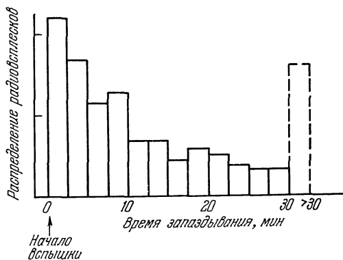
Рис. 29. Распределение числа радиовсплесков III типа относительно начала хромосферных вспышек.
