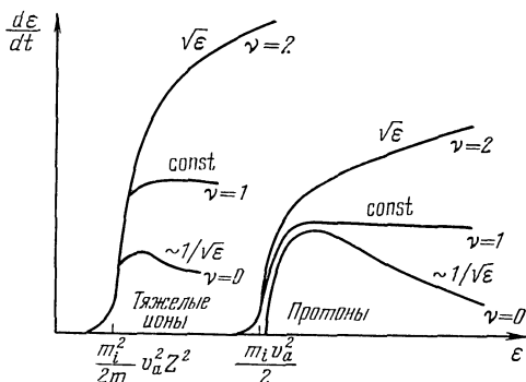
Рис. 11. Ускорение нерелятивистских ионов альвеновскими волнами со спектром W_{\omega}^a = \text{const}/\omega^{\nu} при разных значениях показателя \nu .
