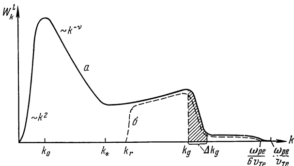
Рис. 1. Спектр ленгмюровской турбулентности: а) случай слабого радиационного затухания или затухания из-за столкновений; б) случай сильного радиационного затухания в области дифференциальной перекачки.
