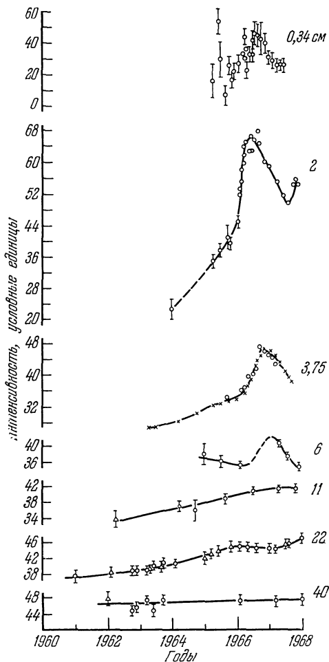
Рис. 44. Изменение спектральной интенсивности излучения на разных длинах волн (в см) со временем для наиболее близкого квазара 3C 273.
