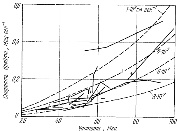
Рис. 31. Зависимость скорости дрейфа радиовсплесков II типа от частоты. Сплошные линии отвечают измерениям скорости дрейфа на нескольких частотах для отдельных радиовсплесков, крестики — измерения на одной частоте; штриховые линии — кривые изменения скорости дрейфа при постоянной скорости движения источника излучения (например, ударной волны).
