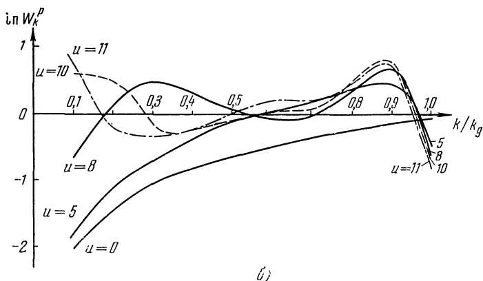
Рис. 39. Спектральные плотности энергии турбулентности продольных (а) и поперечных (б) плазмонов для случая дифференциальной перекачки турбулентности, возбужденной пучком с v_0 = v_{Te}^2/3v_{Ti} для разных моментов времени u = 2\gamma t .
