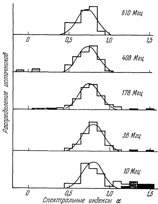
53. Распределение радиисточников по спектральным индексам (на разных частотах).
