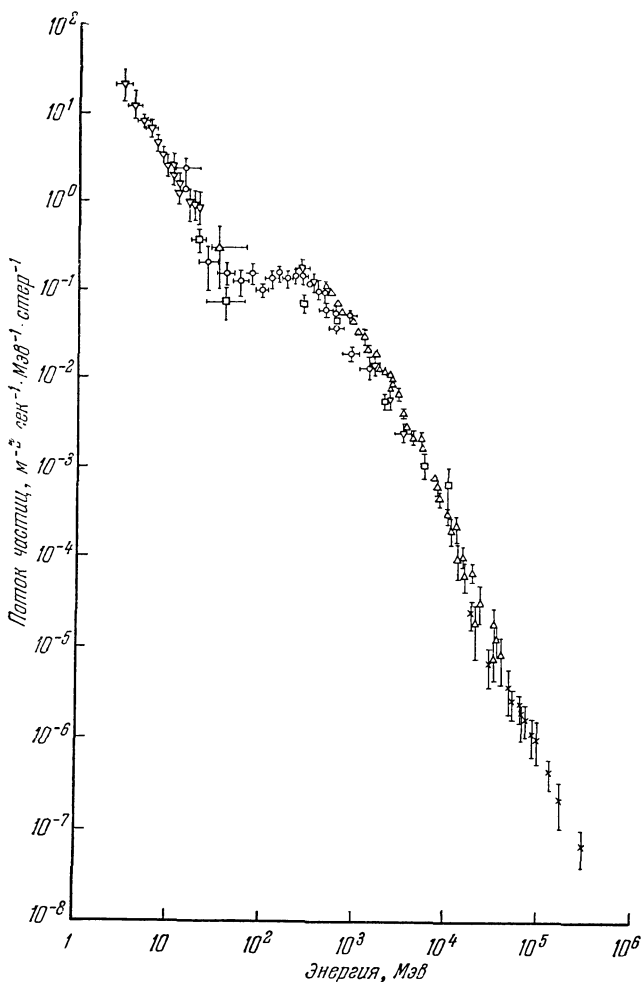
Рис. 82. Наблюдаемый спектр энергий электронной компоненты космических лучей больших энергий.
