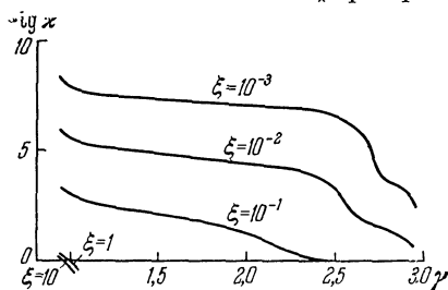
Рис. 63. Зависимость показателя функции распределения \gamma от \xi = \omega_{He}/\omega_{pe} и x = Wl/n_e m_e c^2 .
