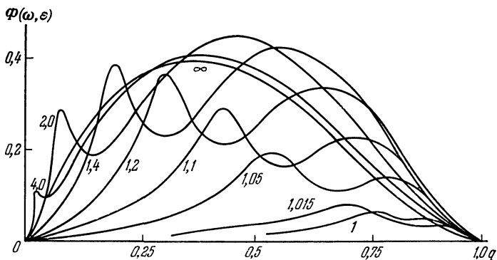
Рис. 61. Спектр излучения при комптоновском рассеянии ленгмюровских волн с v_p \ll c на релятивистских частицах. По оси абсцисс отложена величина q = (\omega/2k_1 c) (m_e c^2/\varepsilon)^2 , числа у кривых — величины \varepsilon/m_e c^2 .
