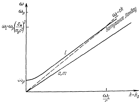
Рис. 76. Дисперсионные кривые для низкочастотных волн ( \omega \ll \omega_H ) в очень сильном магнитном поле. Случай распространения волн вдоль магнитного поля ( \vartheta \ll m_e c^2 / \varepsilon_+ )
