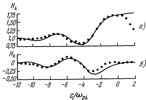
Рис. 20. Осцилляторная структура магнитного поля в ударной волне с числом Маха M = 2 ( n_e = 2 \cdot 10^{14} \text{ см}^{-3} ). Расстояние отсчитывается от фронта ударной волны в единицах c/\omega_{pi} , H —в единицах величины поля перед фронтом волны: а) компонента поля, перпендикулярная к скорости волны; б) компонента поля вдоль скорости
