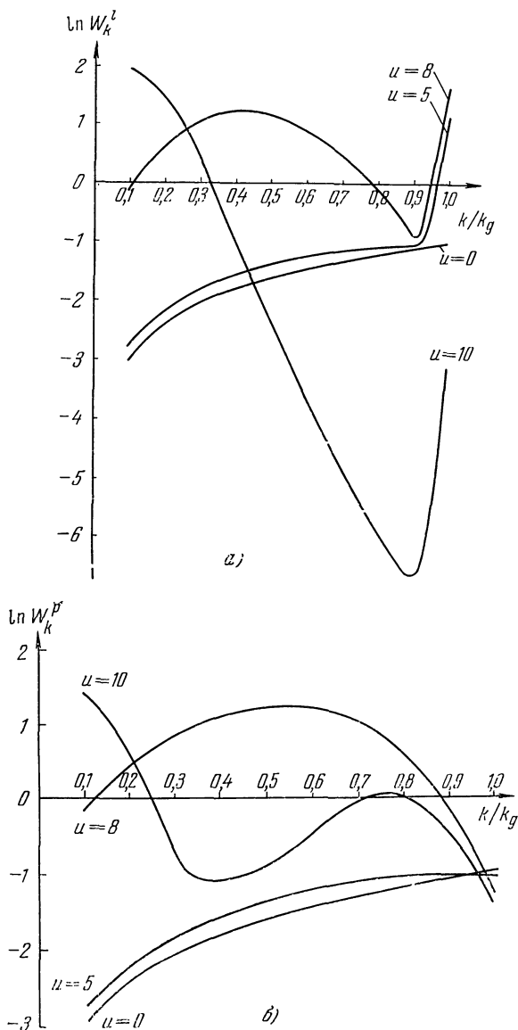
Рис. 40. То же, что и на рис. 39, но для больших скоростей пучка v_0 = v_{Te}/v_{Ti} на границе между областями дифференциальной и интегральной перекачки турбулентности.
