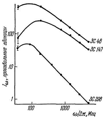
Рис. 52. Спектры радиогалактик. Случай завала спектра на низких частотах.
