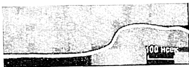
Рис. 18. Профиль фронта бесстолкновительной ударной волны в водородной плазме ( n_e = 5 \cdot 10^{13} \text{ см}^{-3} ).
