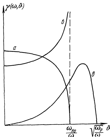
Рис. 78. Зависимость коэффициентов реабсорбции от угла волновым вектором и магнитным полем: а) циклотронное рассеяние при малых частотах, б) магнито-тормозное излучение, в) рассеяние на больших частотах.
